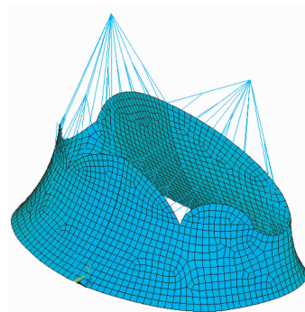
图 3 二尖瓣网格模型
