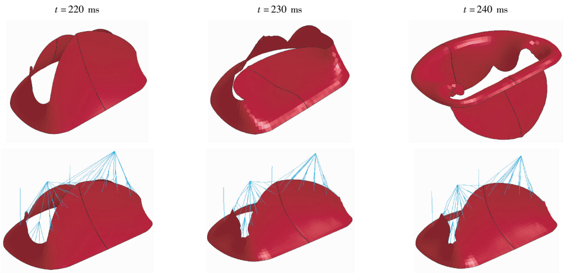
图8 有、无腱索两种情况下瓣叶随时间运动时的位移变化
