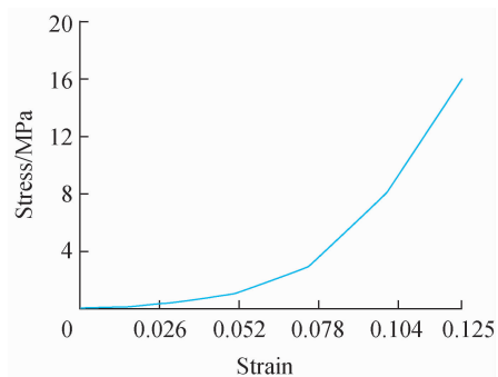
图 4 腱索材料的应力-应变曲线
