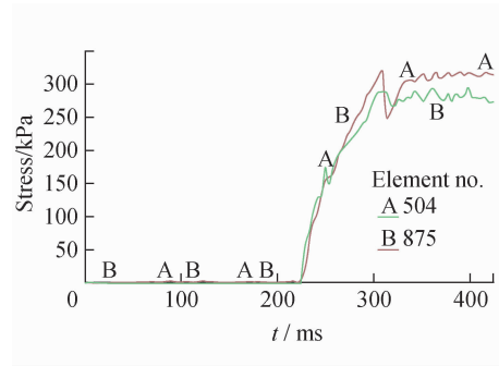
(b) Von Mises 应力随时间变化曲线
